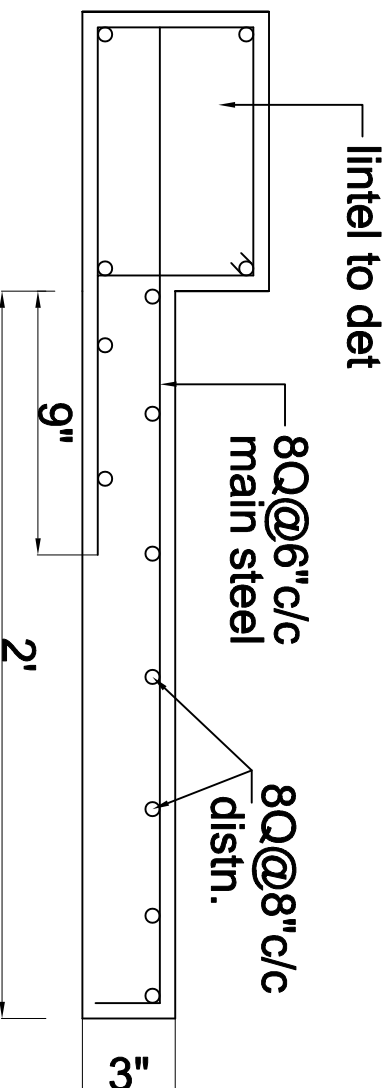
TYP LOFT DET
