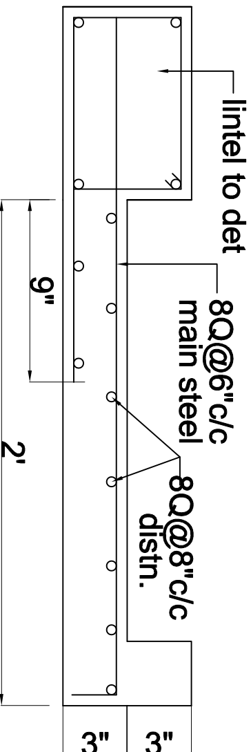
TYP CHEJJA DET
